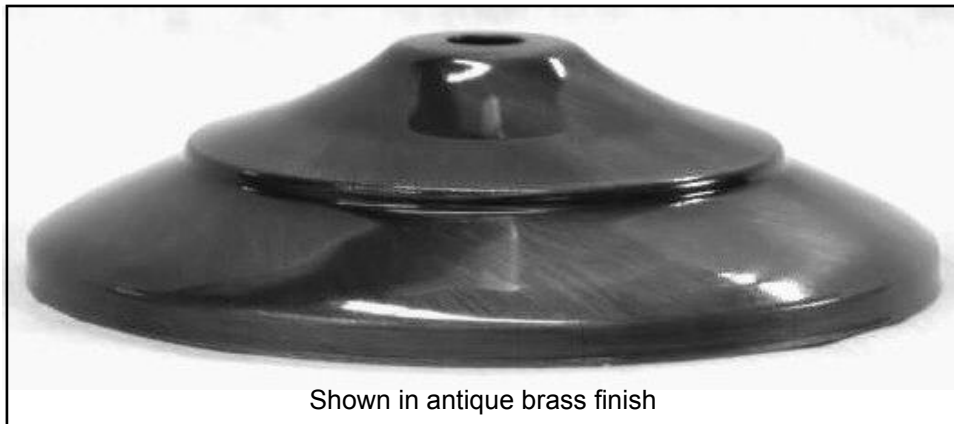
760 5 1/2" OD 1 1/8" high
