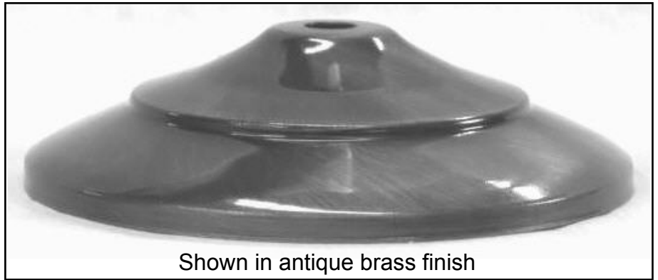
730 5 1/4" OD 1 1/8" high
